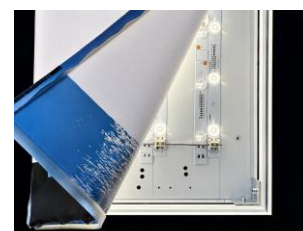
Rahmenaufbau mit LEDs und Stoffbanner
