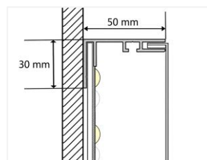
Schichtaufbau: Wand/ Untergrund · Aluminiumprofil mit LED · Wandaufhängung · Stoffbanner mit Keder
