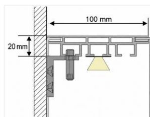
Schichtaufbau: Wand/ Untergrund · Blockout-Textil-Rückwand · Aluminiumprofil mit LED · Wandaufhängung · Stoffbanner mit Keder
