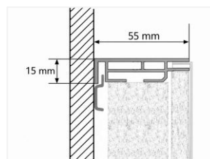
Schichtaufbau: Wand/ Untergrund · Aluminiumprofil · Akustikmaterial · Stoffbanner mit Keder
